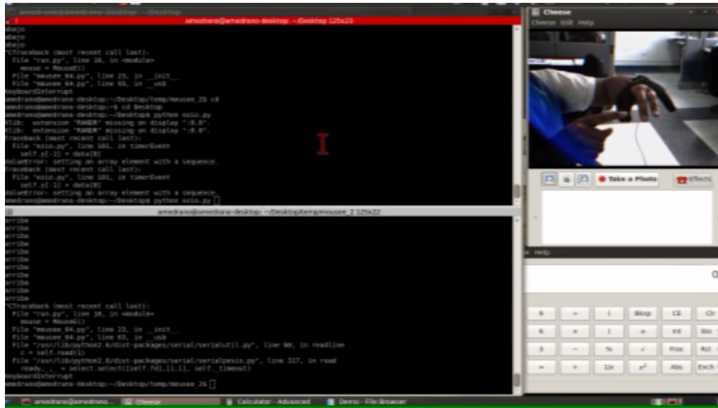
Figura 4: El guante correspondiente al prototipo inicial funcionando bajo el Sistema Operativo GNU/Linux con el entorno GNOME y sensores flexibles resistivos
